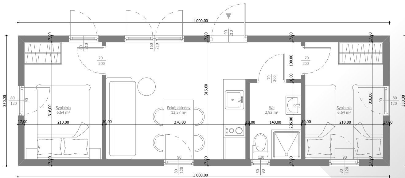
PŮDORYS
